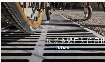
在室外下水道口，将孔洞宽度设计不大于 1.3cm，条状空洞垂直于通行方向，减少意外发生
